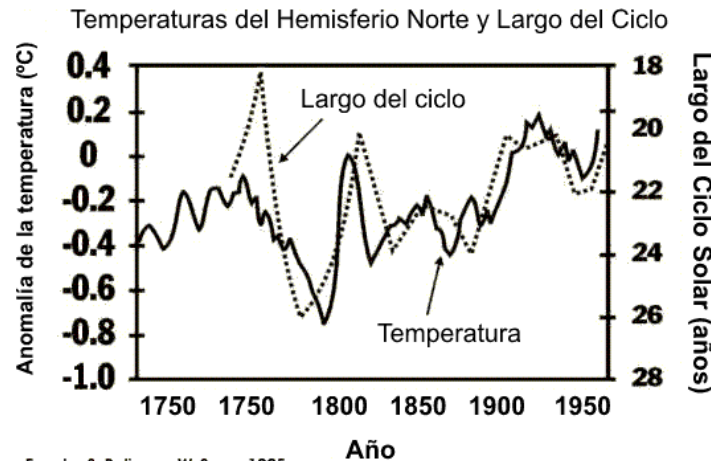
Figura 3: Relación entre Ciclos Solares y Temperatura
