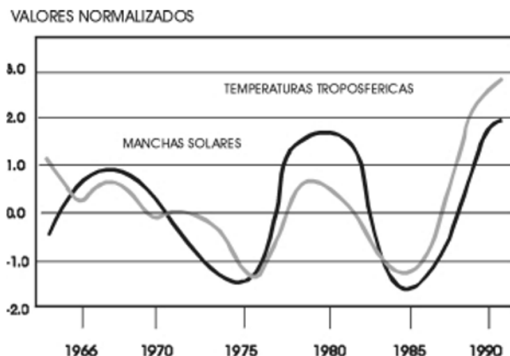
Fig. 4. Variación de promedios anuales del número de manchas solares y las temperaturas troposféricas en latitudes medias del Hemisferio Norte entre 1966 y 1990. El coeficiente de correlación entre los conjuntos de datos es r = 0.76
