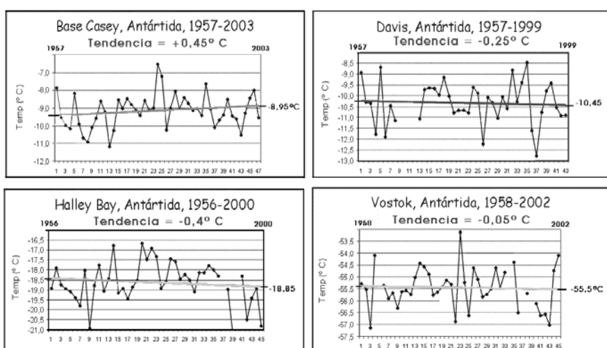
Figura 2: Temperaturas en las estaciones Casey (base Antártica de Australia), Davis, Halley Bay, y Vostok.
